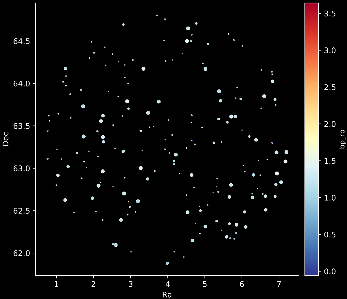
APOGEE DR17 Field: [CVZTILE_093+32_btx] Stars: 184
