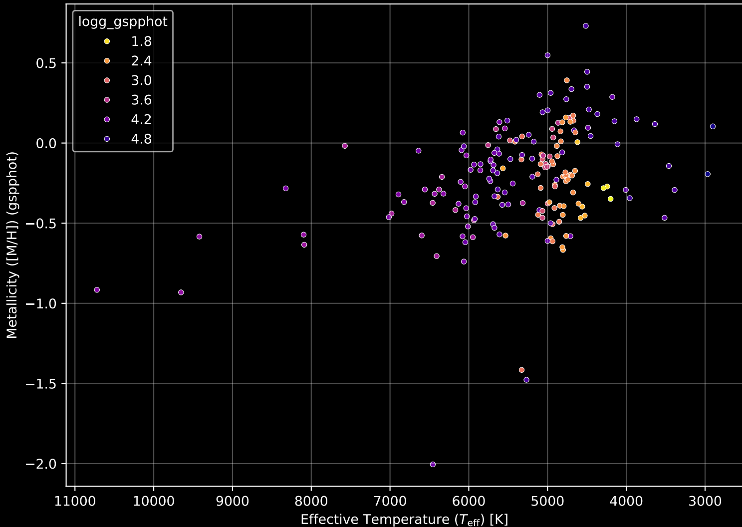
APOGEE DR17 Field: [CVZTILE_093+32_btx] Stellar Population Parameters (n= 184)
